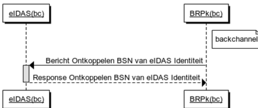
Figuur 4: Cyclus van Ontkoppelvezoek
