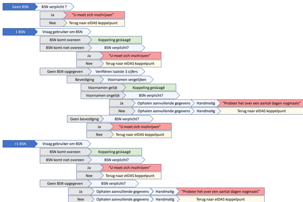
Figuur 2: Verwerken zoekvraag
