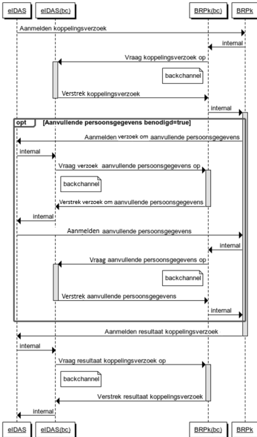
Figuur 3: Cyclus van Koppelingsverzoek
