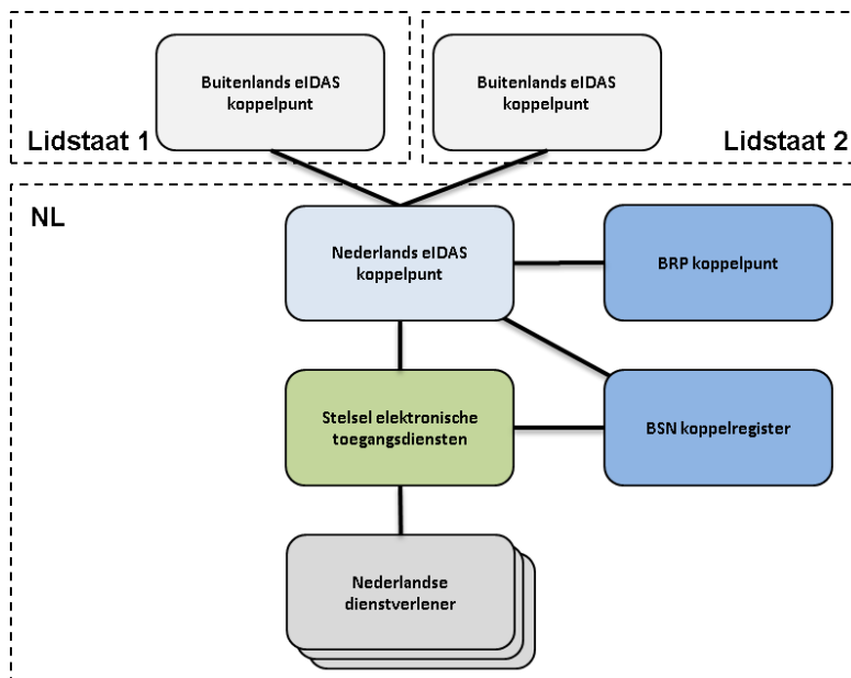
Figuur 1: Context BRP-Koppelpunt
